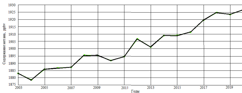
Рис. 5. Изменения содержания метана в зимний период с 2003 по 2019 годы по территории Казахстана.
