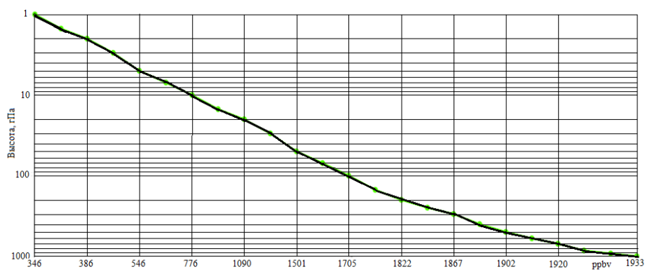
Рис. 4. Среднее вертикальное распределение метана по территории Казахстана за 2019 год.
