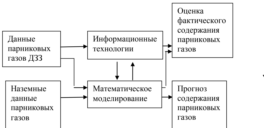
Рис. 1. Структура космического мониторинга парниковых газов.
