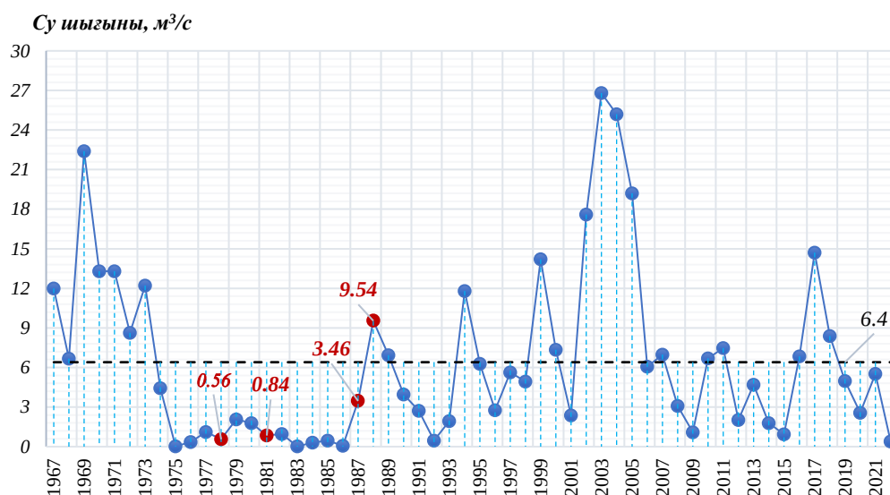
Сурет 4. Шу өзенінің Кіші Арна – Уланбел учаскесі бойынша қалпына келтірілген орташа жылдық су шығындары (1967...2022 жж.)
