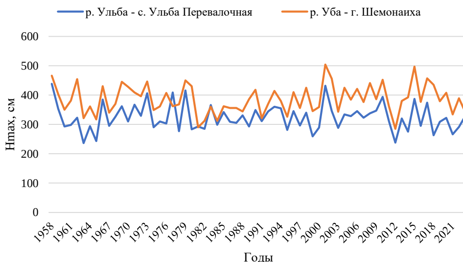
Рисунок 4. Динамика максимальных уровней воды на реках Ульба и Уба
