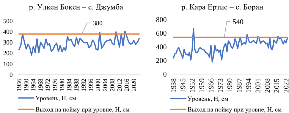
Рисунок 6. Динамика максимальных уровней воды с указанием отметки выхода на пойму
