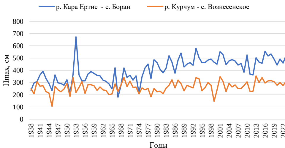
Рисунок 5. Динамика максимальных расходов воды на реках Кара Ертис и Курчум
