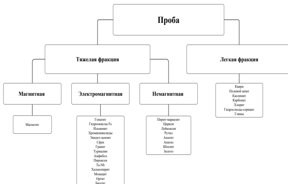
Рисунок 1. Минералы тяжелой и легкой фракции шлиховых проб обогащённого керна на месторождении урановой промышленности РК
