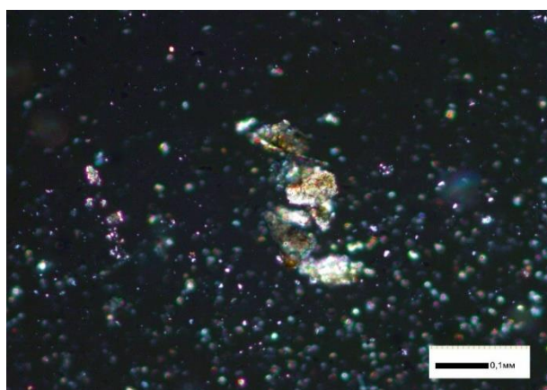
Рисунок 2. Сфен бурый (увеличение 100-ное в иммерсии)
