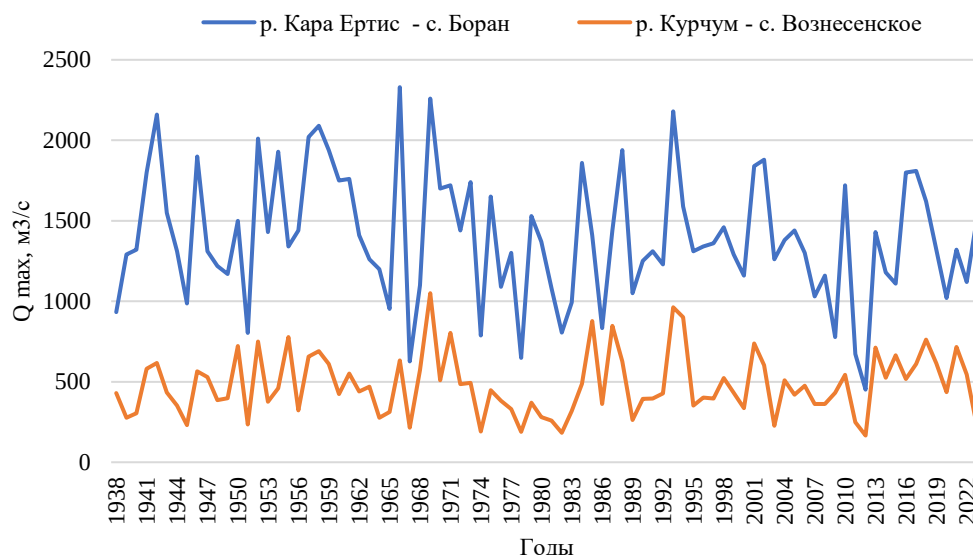
Рисунок 3. Динамика максимальных расходов воды на реках Кара Ерчис – с. Боран и Курчум – с. Вознесенское
