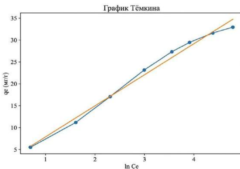
Рисунок 12. График Темкина в координатах q_e - \ln C_e
