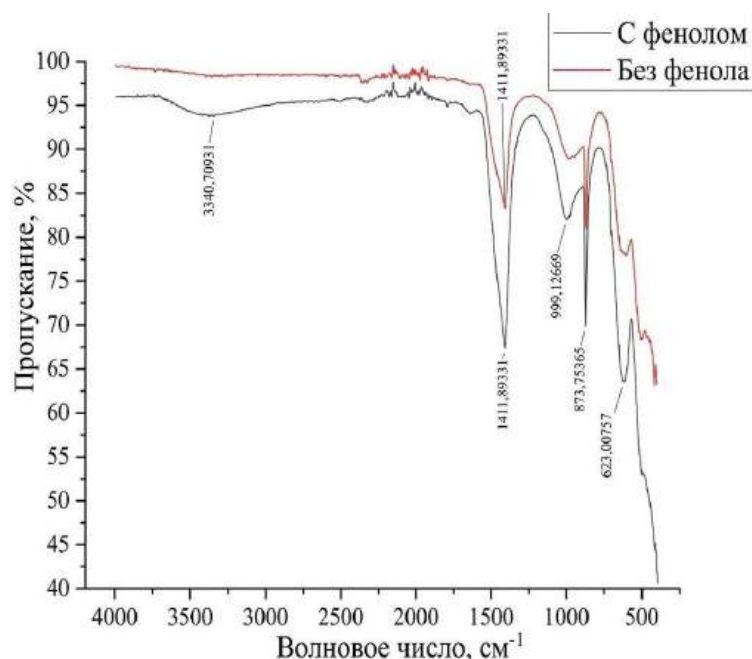
Рисунок 5. ИК-спектры модифицированного шлама (АМ-01) до и после адсорбции фенола
