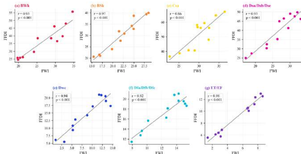
Рисунок 10. Графики рассеяния значений FWI и FFDI (среднесуточные значения по зоне, n = 12 ) для семи климатических зон Кеппена-Гейгера территории Казахстана за период 20...31 июля 2025 г.: (а) пустыня/полупустыня (BWk); (б) степь (BSk); (в) умеренный тёплый (Csa); (д) континентальный с сухим летом (Dsa/Dsb/Dsc); (е) континентальный с сухой зимой (Dwc); (ф) континентальный влажный (Dfa/Dfb/Dfc); (г) высокогорный/тундровый (ET/EF). r – коэффициент корреляции Пирсона; p – уровень статистической значимости
