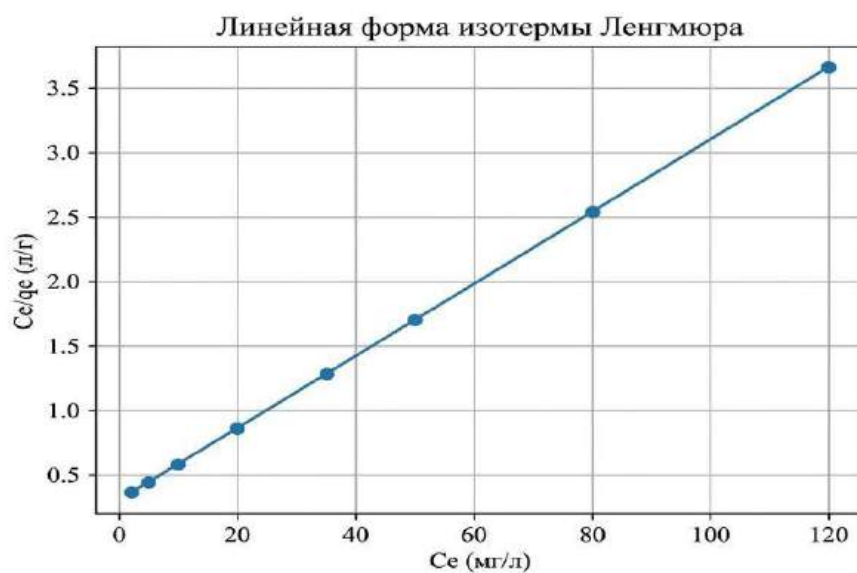
Рисунок 10. Линеаризованный график Ленгмюра
