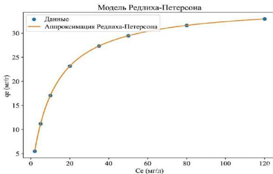
Рисунок 13. Нелинейная аппроксимация по модели Редлиха-Петерсона
