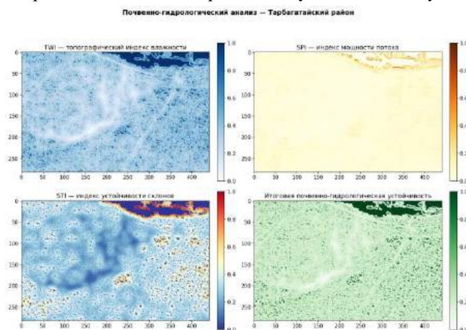
Рисунок 1. Карты топографических индексов влажности и эрозионной устойчивости исследуемой территории
