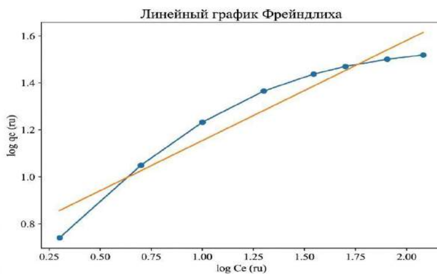
Рисунок 11. Линеаризованный график Фрейндлиха
